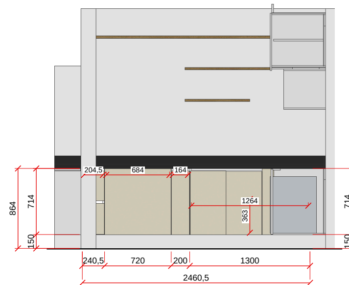
VISTA B - ESC. 1:40
