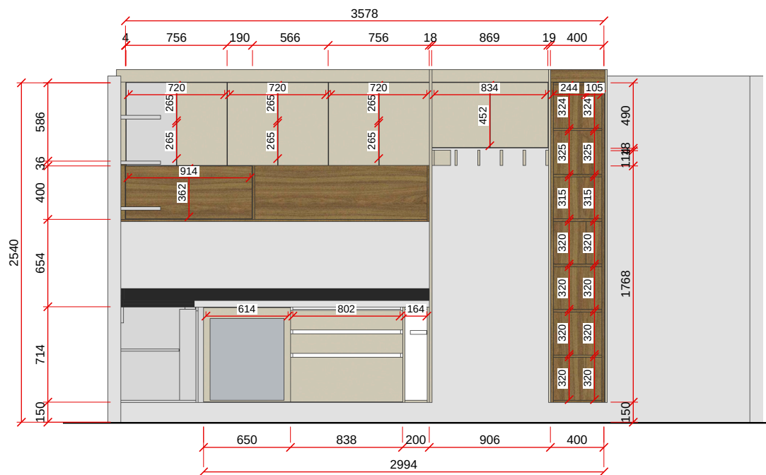
VISTA A - ESC. 1:40
